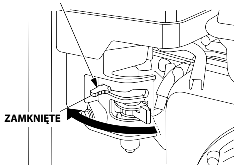
DŹWIGIENKA SSANIA
